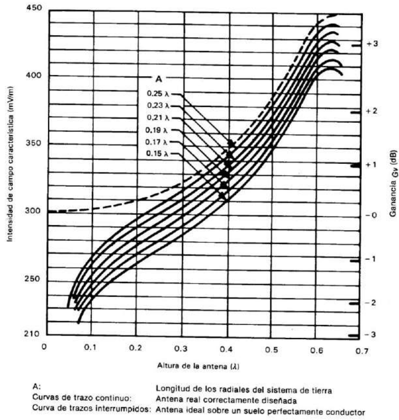
FIGURA 1 – Intensidades de campo características para antenas verticales simples utilizando sistemas de tierra de 120 radiales
