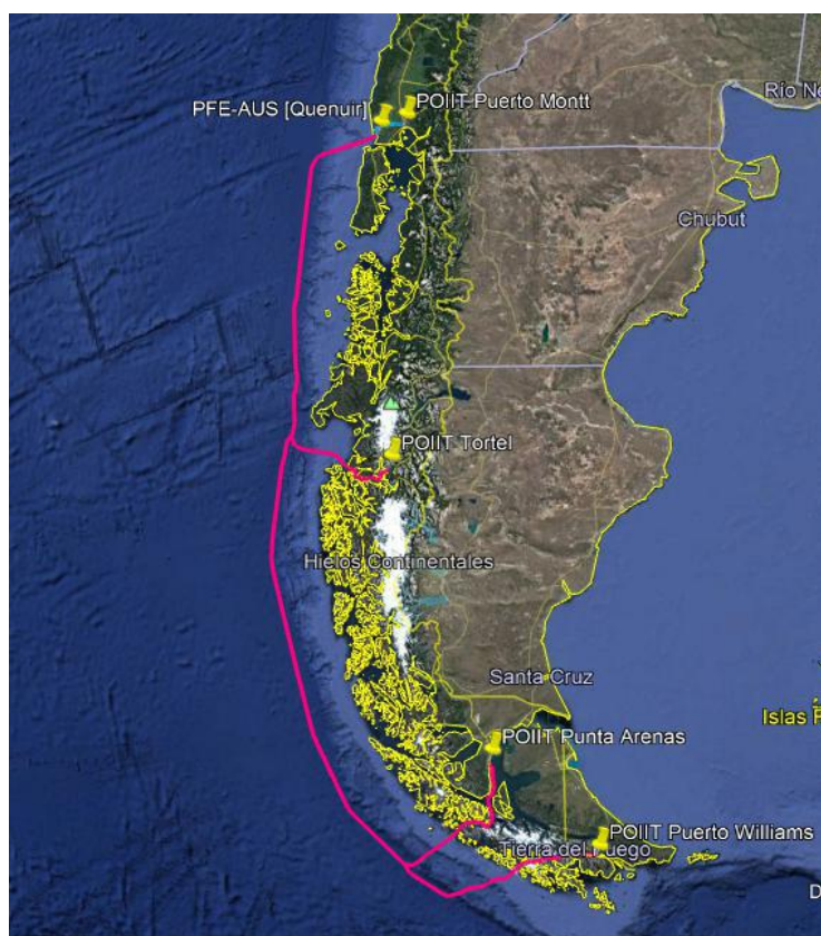
Ilustración 3 - Troncal Submarina FOA
