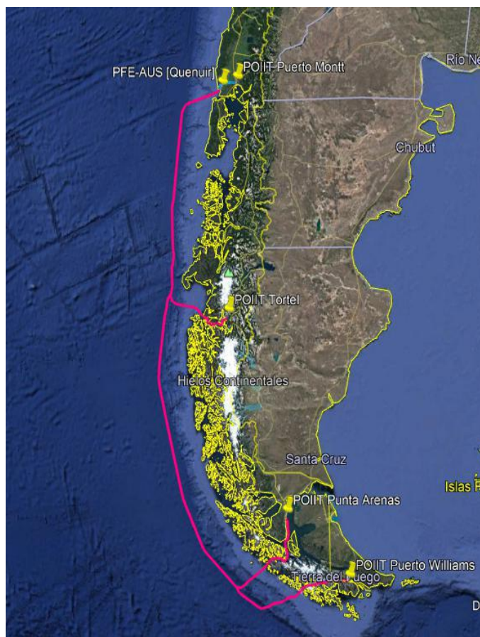
Ilustración 2 – Troncal Submarina FOA
