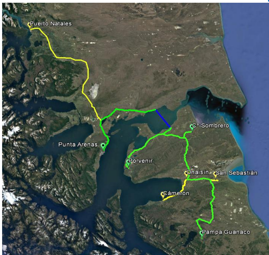
Ilustración 3 - Trazado FOA Magallanes - Conductividad Austral Ltda
