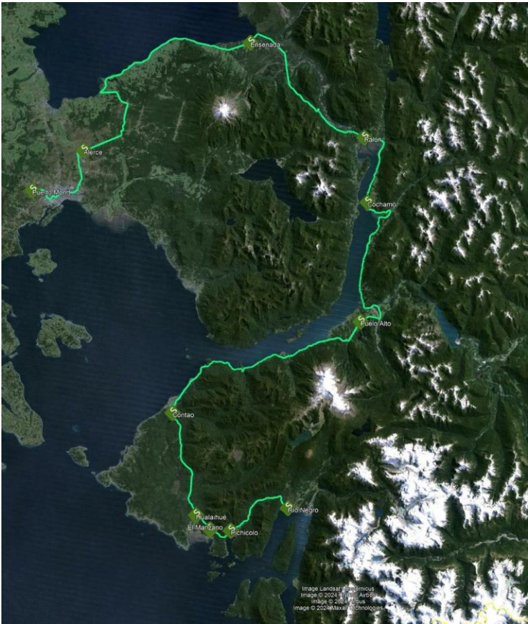
Ilustración 3 - Trazado Troncal Terrestre Los Lagos FOA
