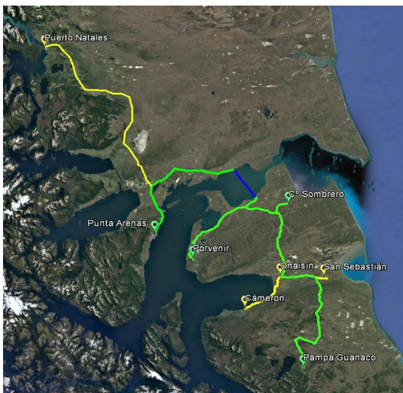
Ilustración 3 – Trazado FOA Magallanes – Conductividad Austral Ltda
