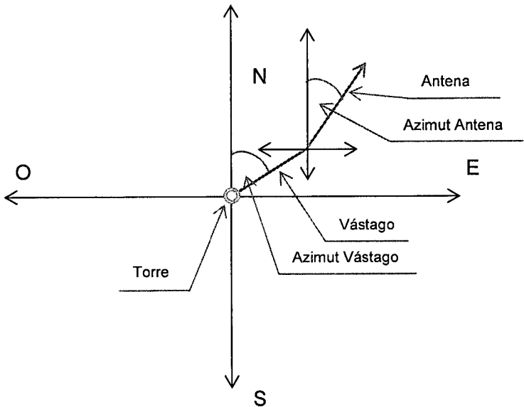
Esquema de configuración vástago, antena.
