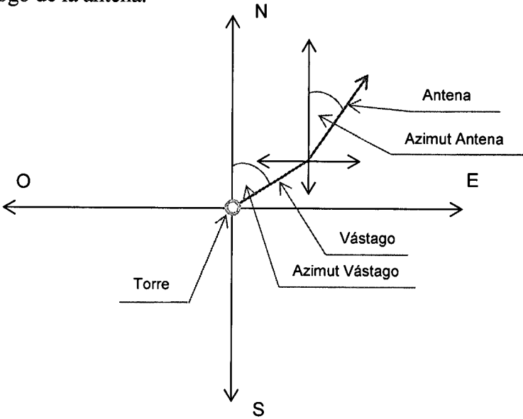
Esquema de configuración vástago, antenna.
